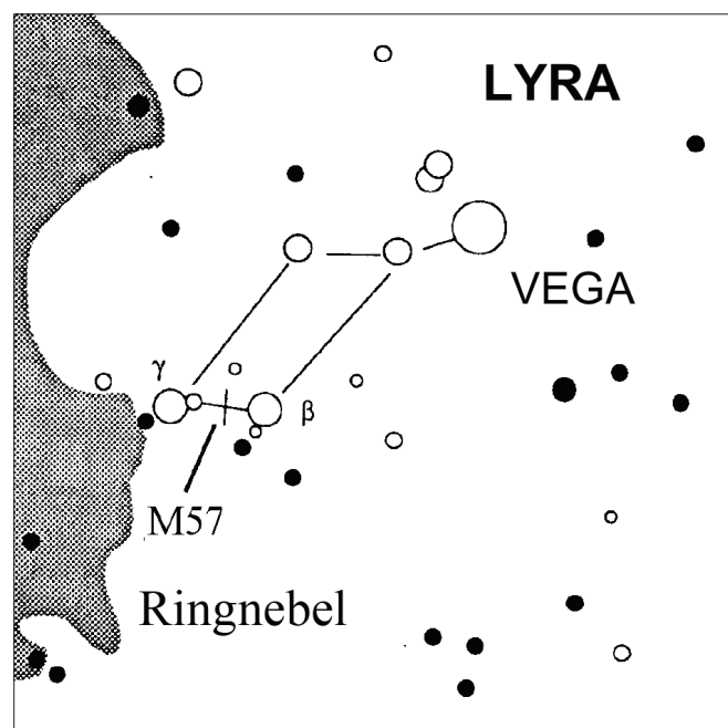
Abb. 17 Ringnebel
